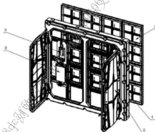
可变情报板组成示意图
