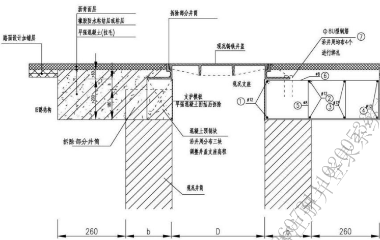
(a) 检查井加固设计图
