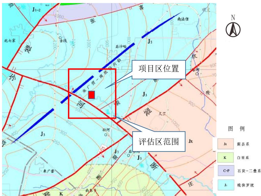
图 3-2 孙河断裂与评估区位置
