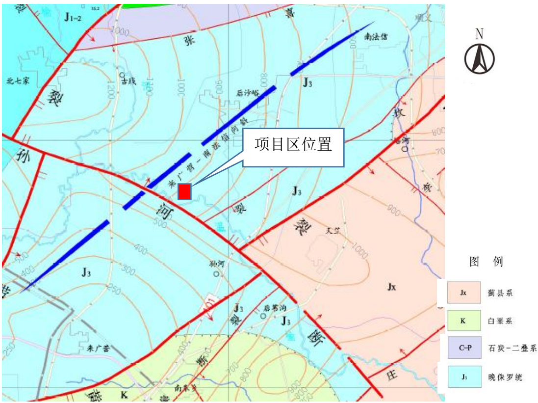
图2-4 评估区基岩地质图
