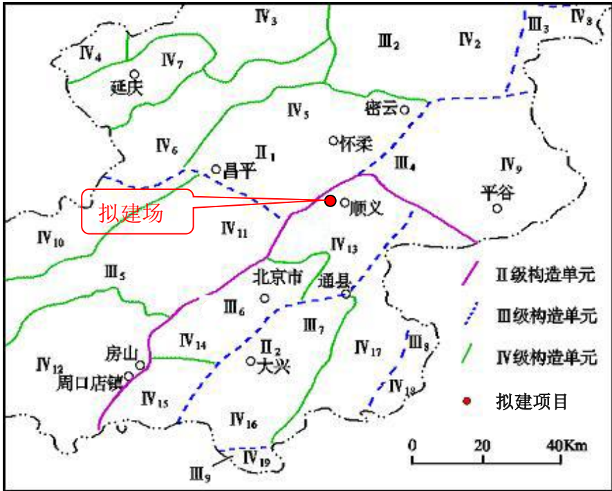
图2-5 拟建项目大地构造位置图
