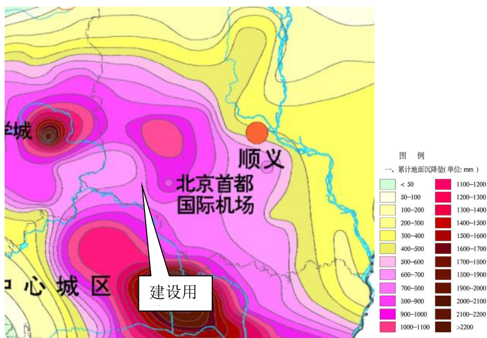
图 3-2 北京市平原地区 1955 年-2021 年累计地面沉降量分区图
