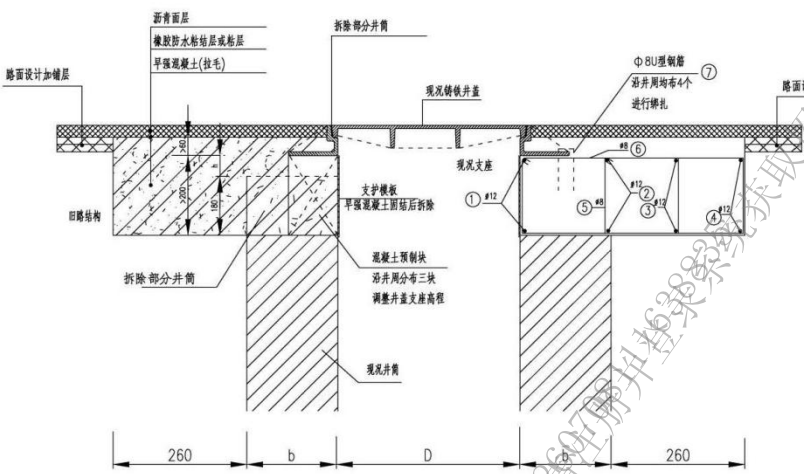
(a) 检查井加固设计图
