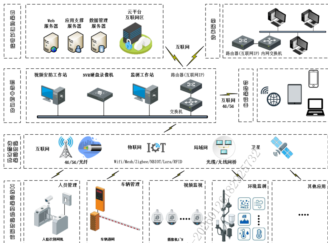
图26-4-2 系统组成及结构示意图
