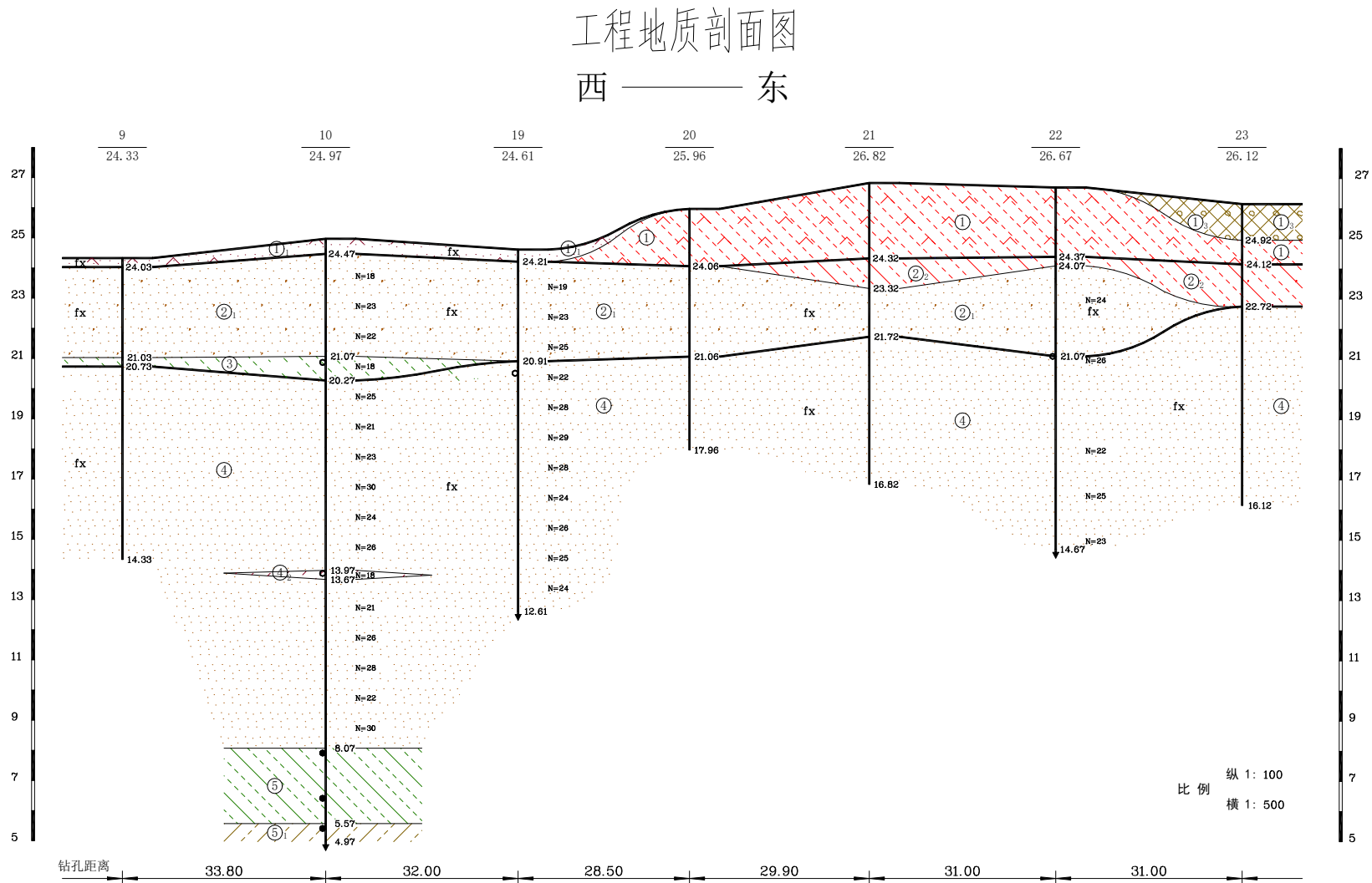
图 2-9 建设用地周边经典地质剖面图（西-东）
