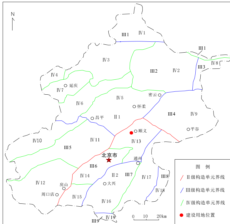
图 2-4 北京市构造分区略图
