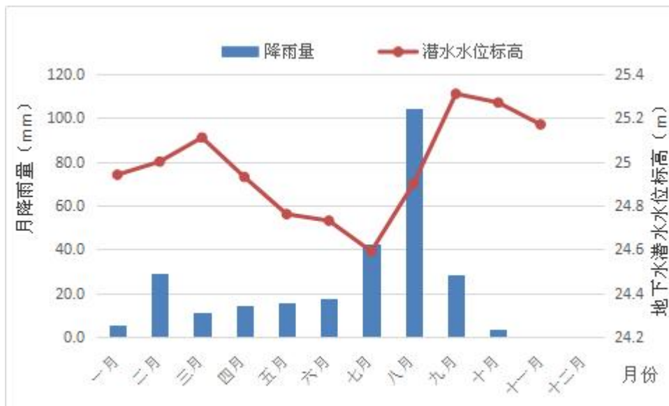
图 2-12 顺义区 2020 年月降水量与南法信监测孔潜水水位动态对比图
