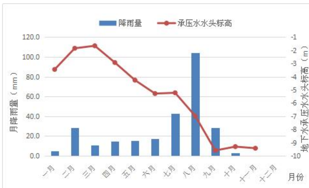
图 2-14 顺义区 2020 年月降水量与南法信监测孔承压水水头动态对比图
