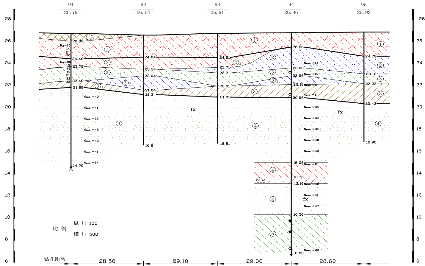
图 2-10 建设用地周边经典地质剖面图 (北-南)
