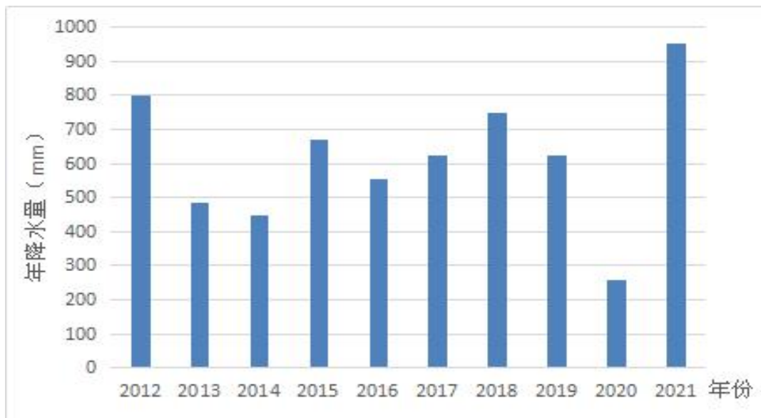
图 2-1 顺义区 2012~2021 年降水量直方图
