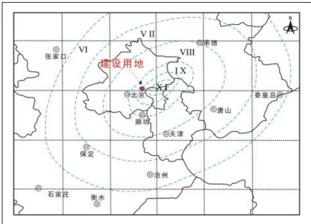
图 2-7 1679 年三河~平谷 8 级地震等震线
