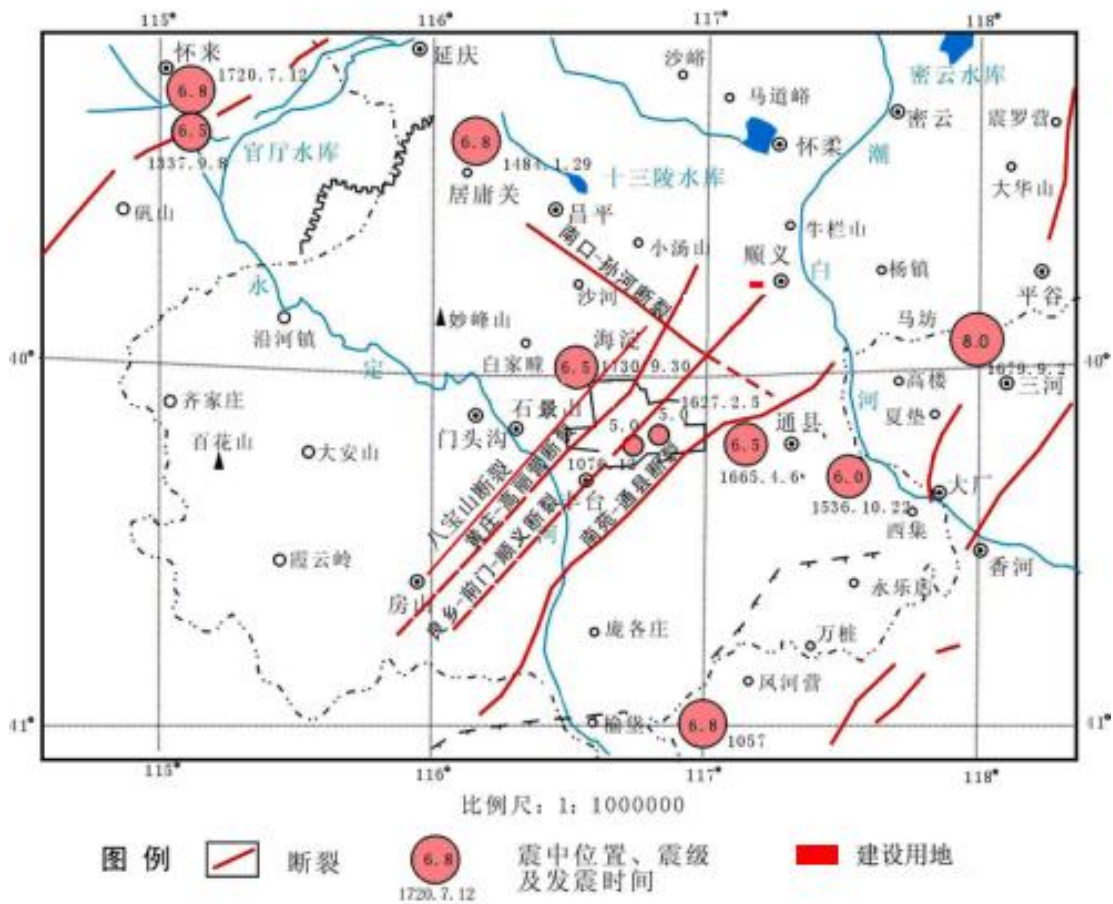
图 2-6 北京市周围历史强震震中分布图
