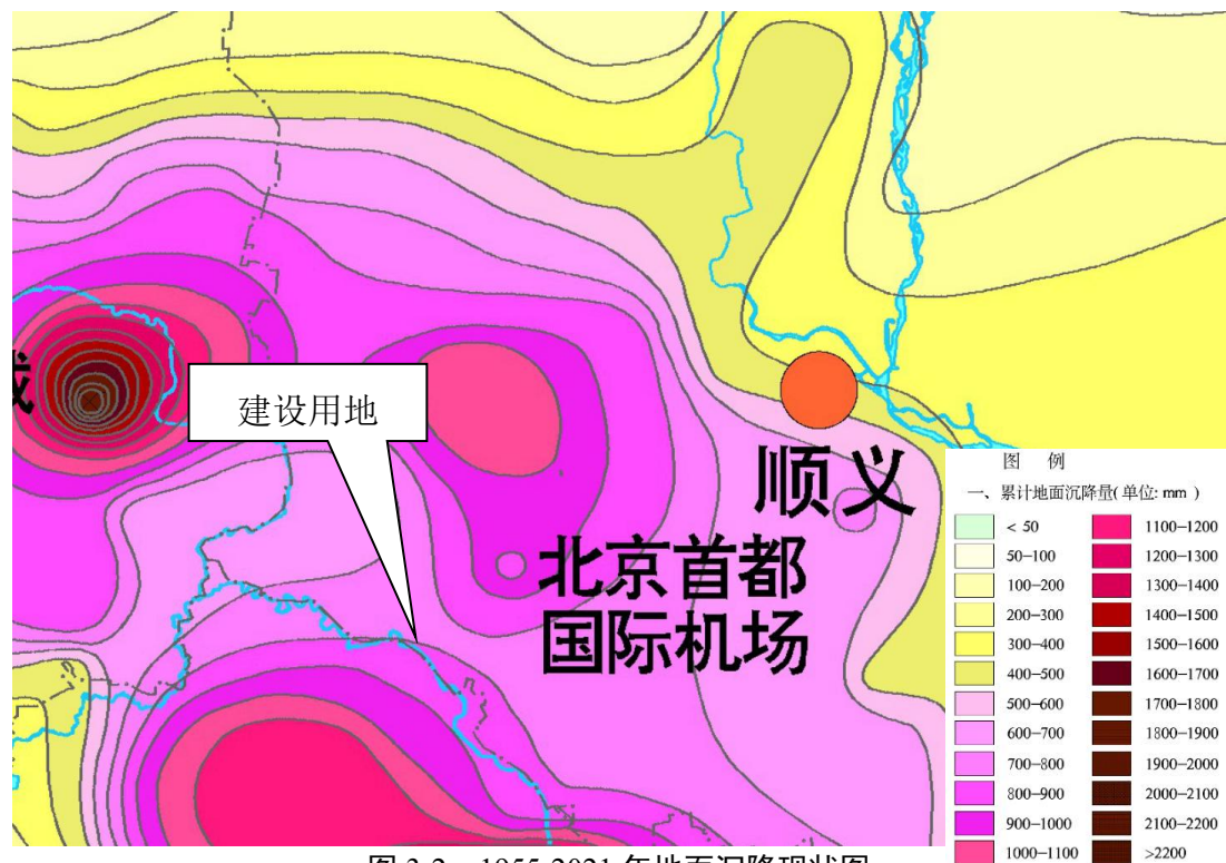
图 3-2 1955-2021 年地面沉降现状图
