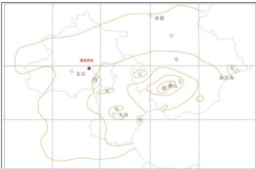
图 2-8 1976 年唐山 7.8 级地震等震线
