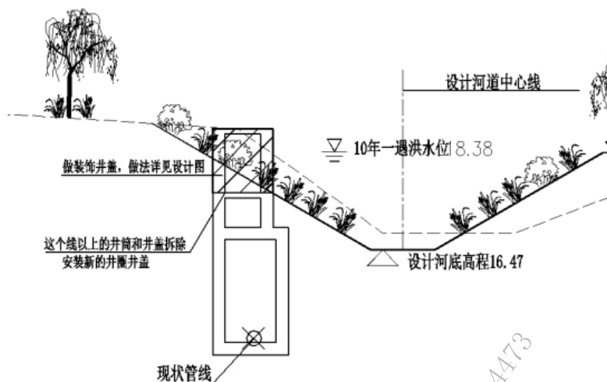
现状检查井改造图
