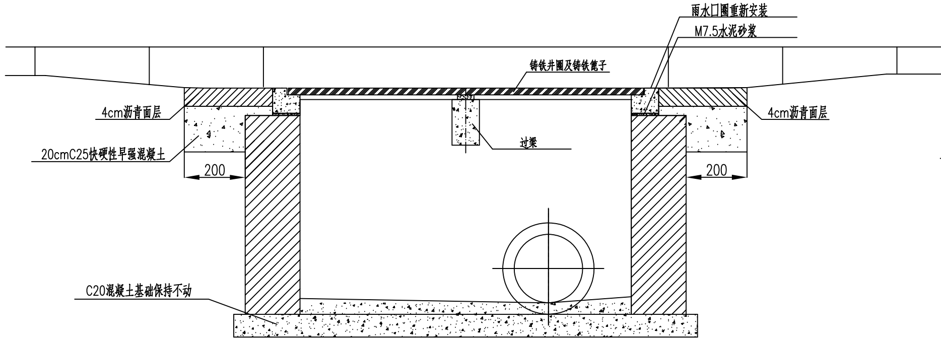
I—I 剖面图
