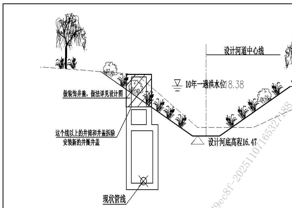
现状检查井改造图
