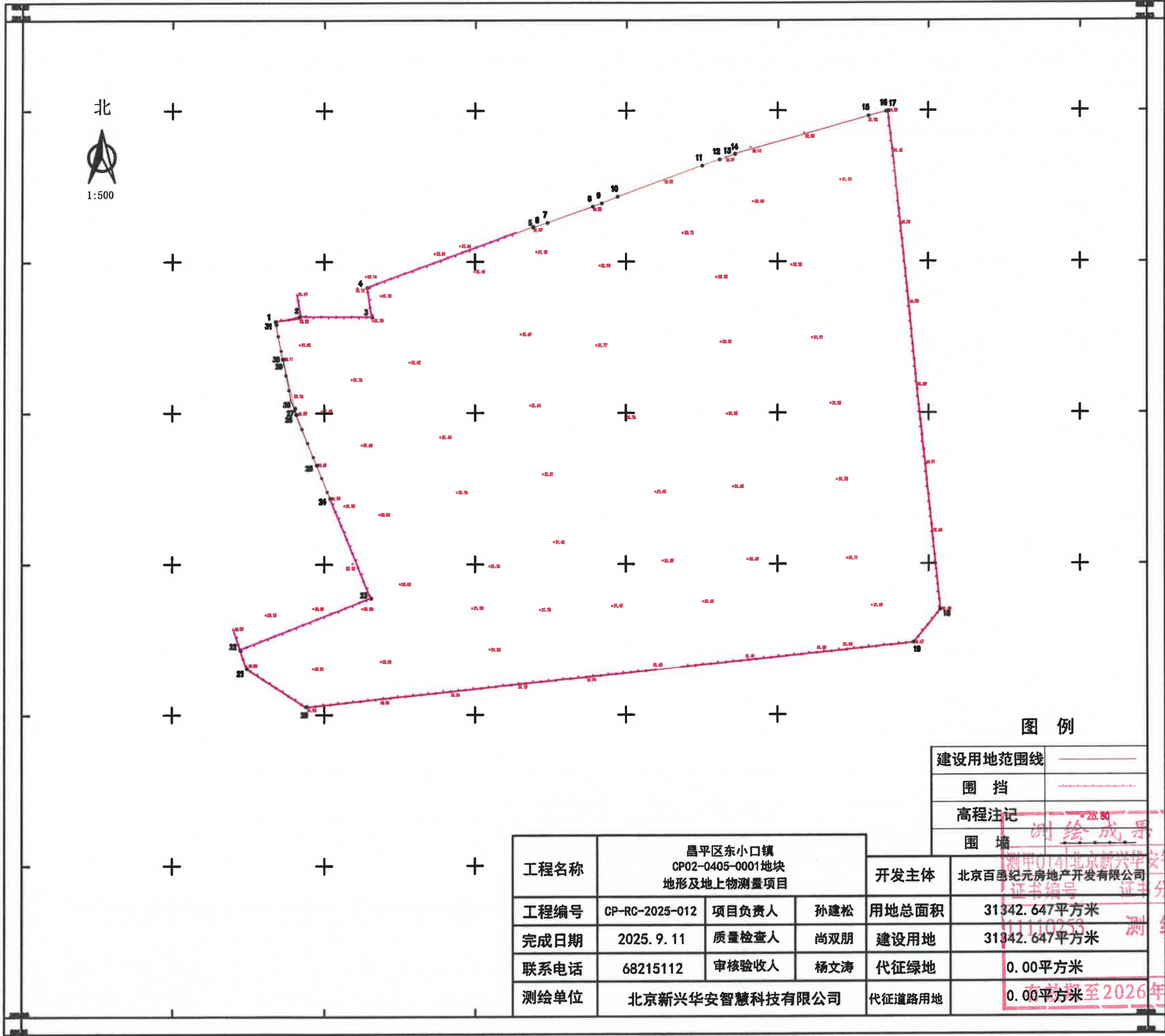
昌平区东小口镇CP02-0405-0001地块地形及地上物测量项目测量平面图
