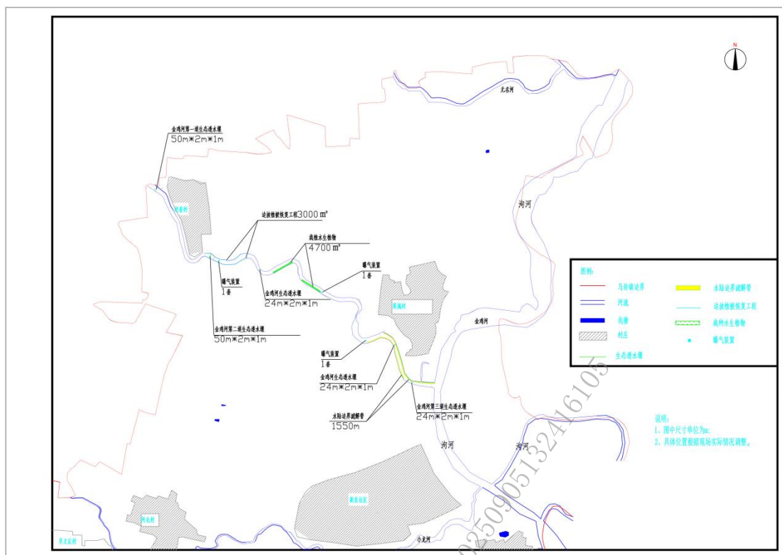
图 4-1 工程布置图
