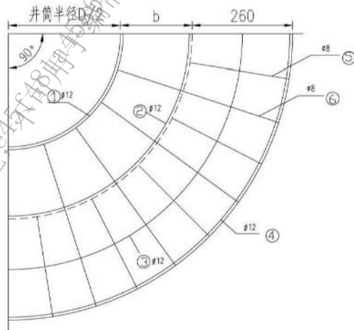
(b) 钢筋布置示意图
