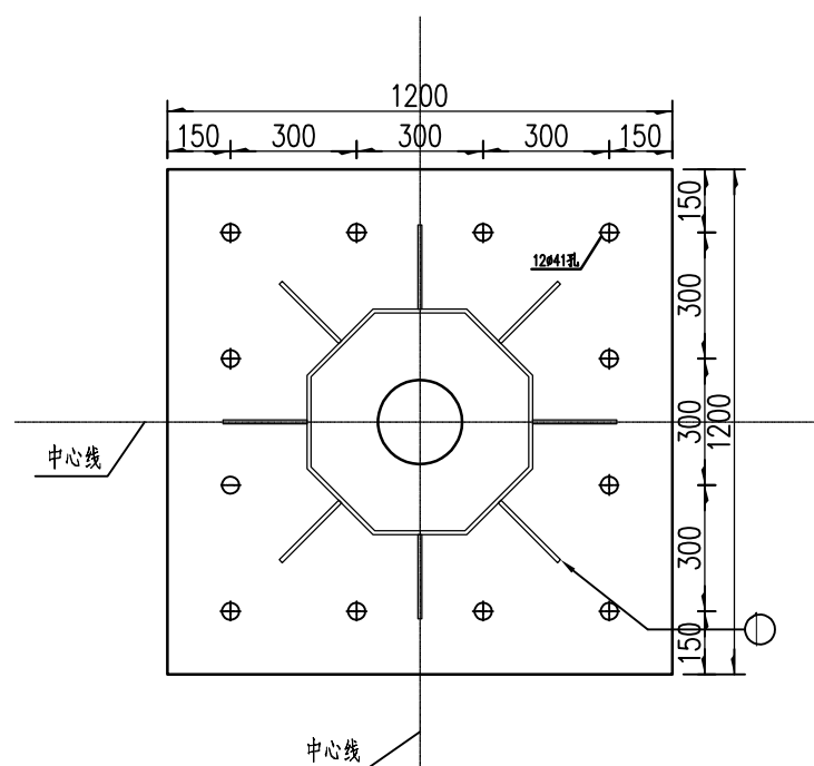
件1 1:12.5 t=8
