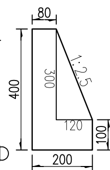
件1 1:12.5 t=8
