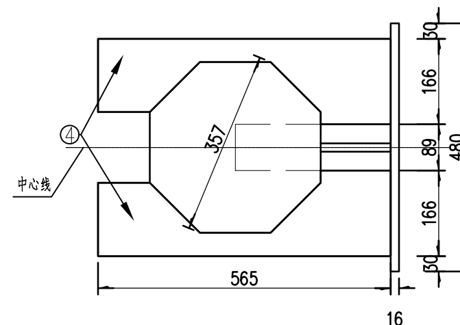
C-C 1:10
