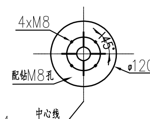
D向 1:5
