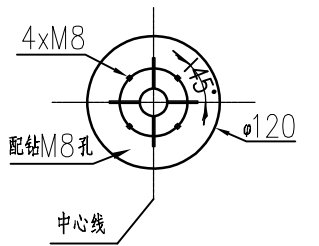
D 向 1:5
