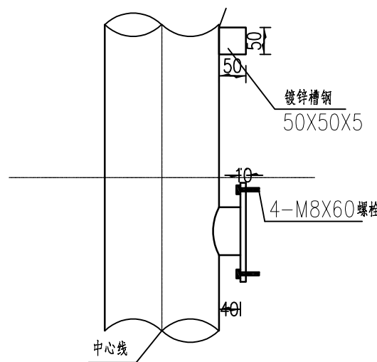
B-B 1:5
