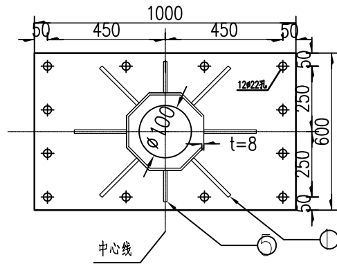
A-A 1:12.5
