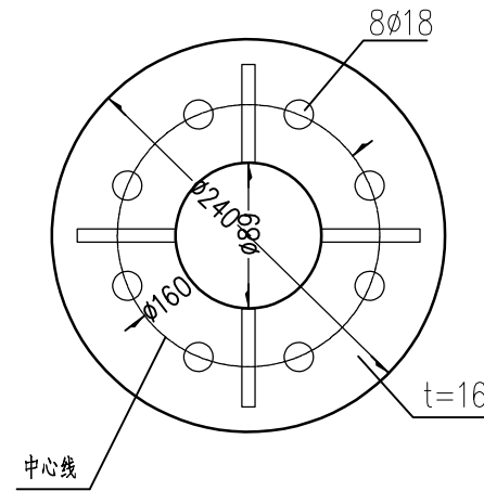
B-B 1:5
