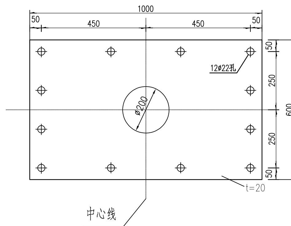
法兰盘大样图 (1:10)
