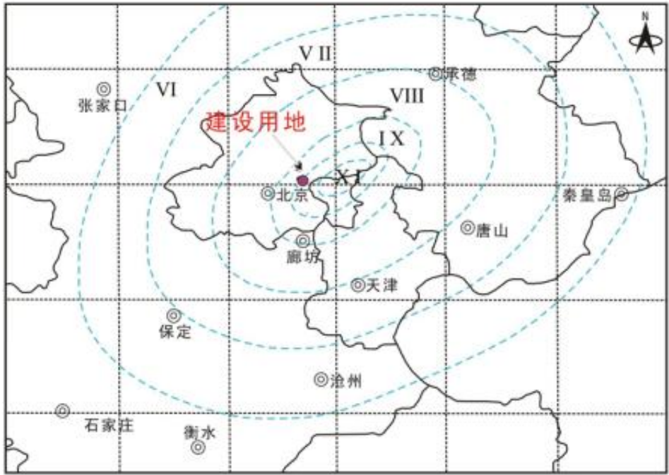
图 2-6 1679 年三河~平谷 8 级地震等震线
