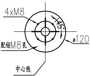
D向 1:5
