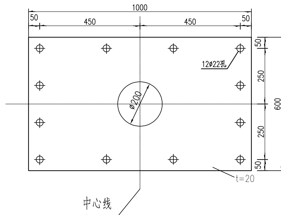
法兰盘大样图 (1:10)
