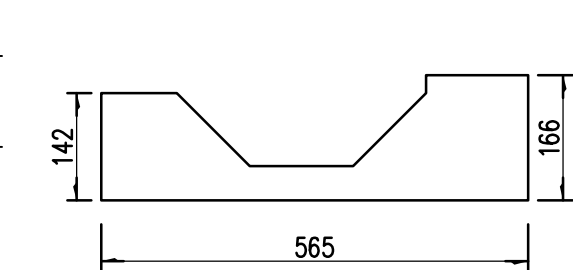
件4 1:5 t=8
