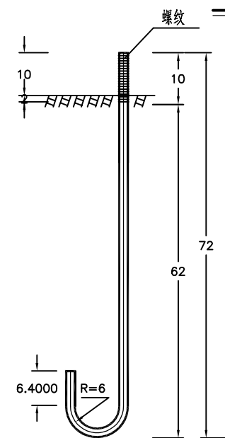
M20地脚螺栓大样图 (L=1100mm)
