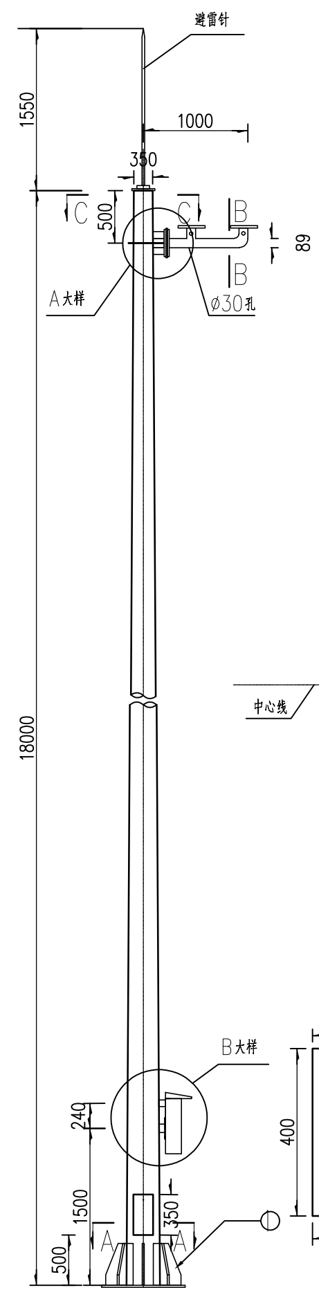
件1 1:12.5 t=8
