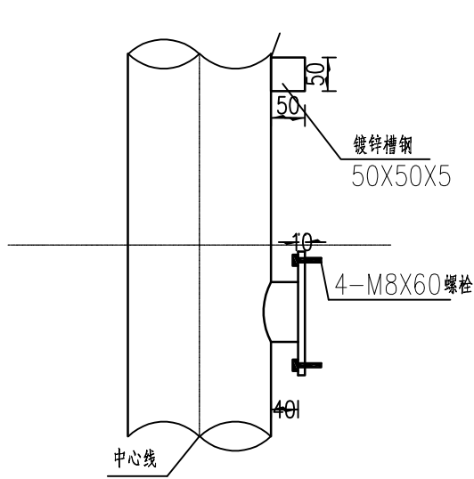
B-B 1:5
