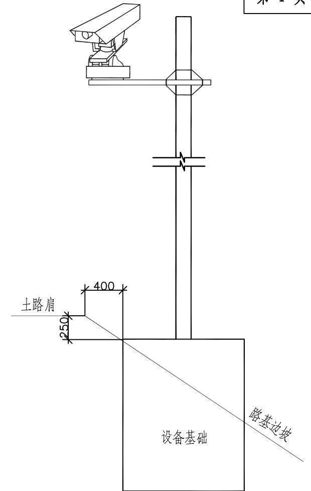
设备基础位置示意图
