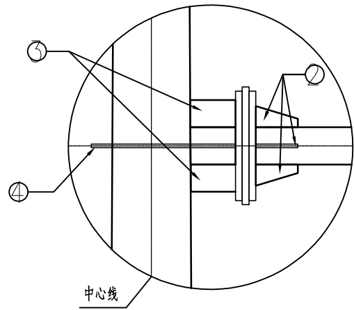
A大样 1:12.5
