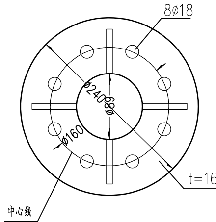
B-B 1:5
