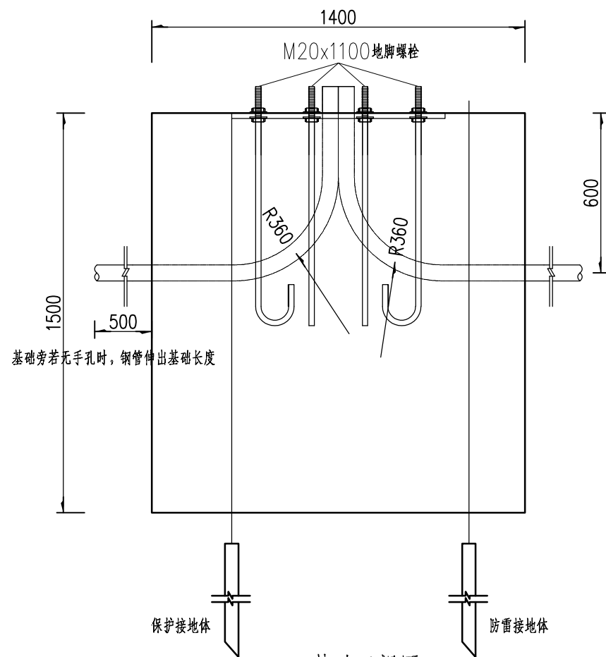
基础正视图 (1:20)
