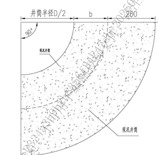
(b) 钢纤维混凝土布置示意图
