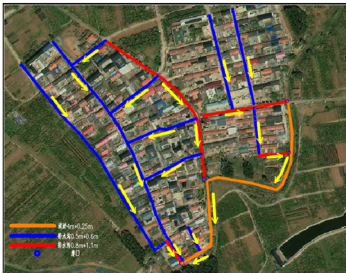
排水工程平面布置示意图
