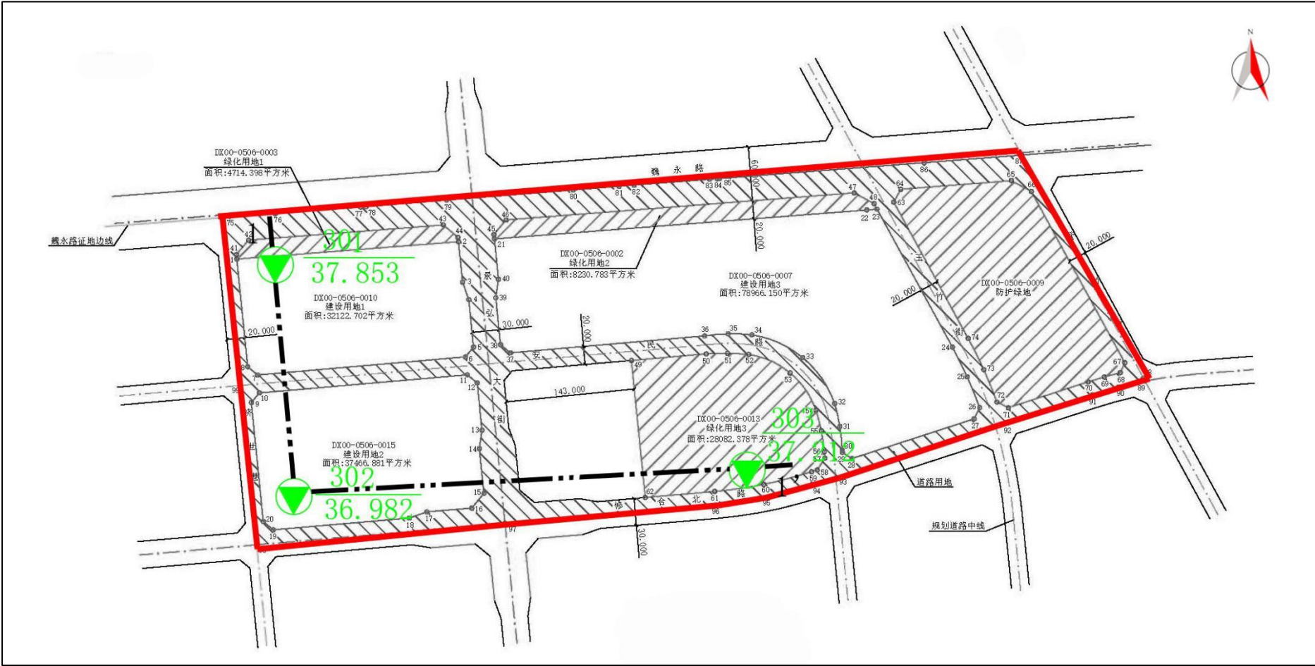
图 2-5 平面布置图
