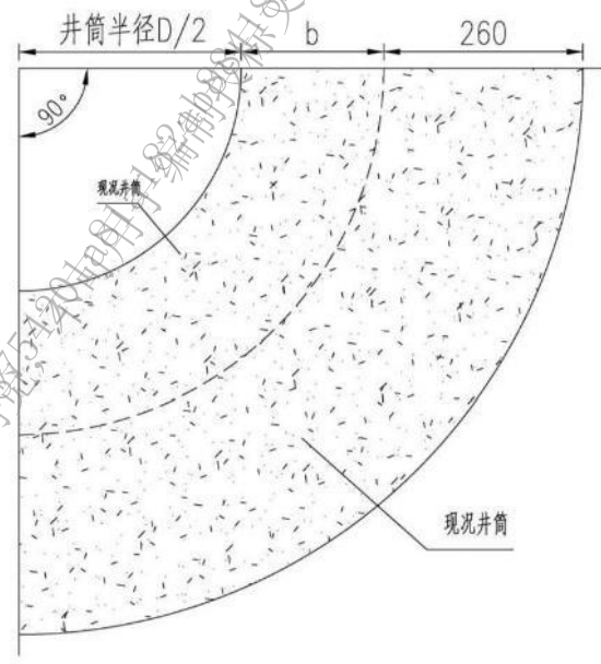
(b) 钢纤维混凝土布置示意图
