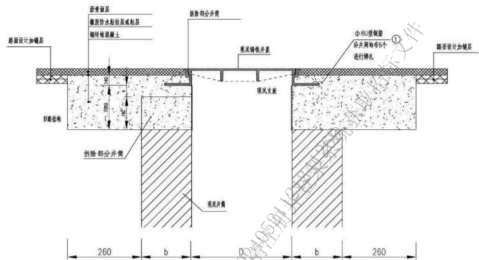
(a) 检查井加固设计图
