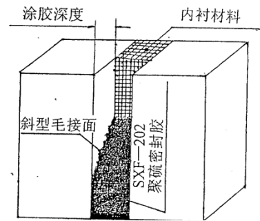
密封胶斜型毛面搭接示意图
