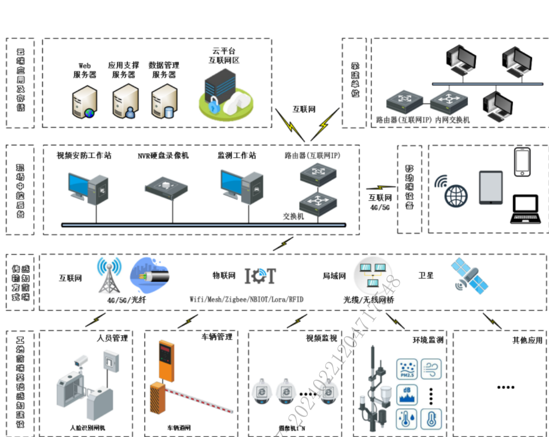
系统组成及结构示意图
