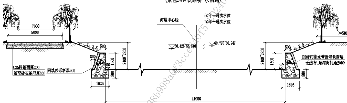
标准横断面图 1:100 (京包24#铁路桥~水南路)
