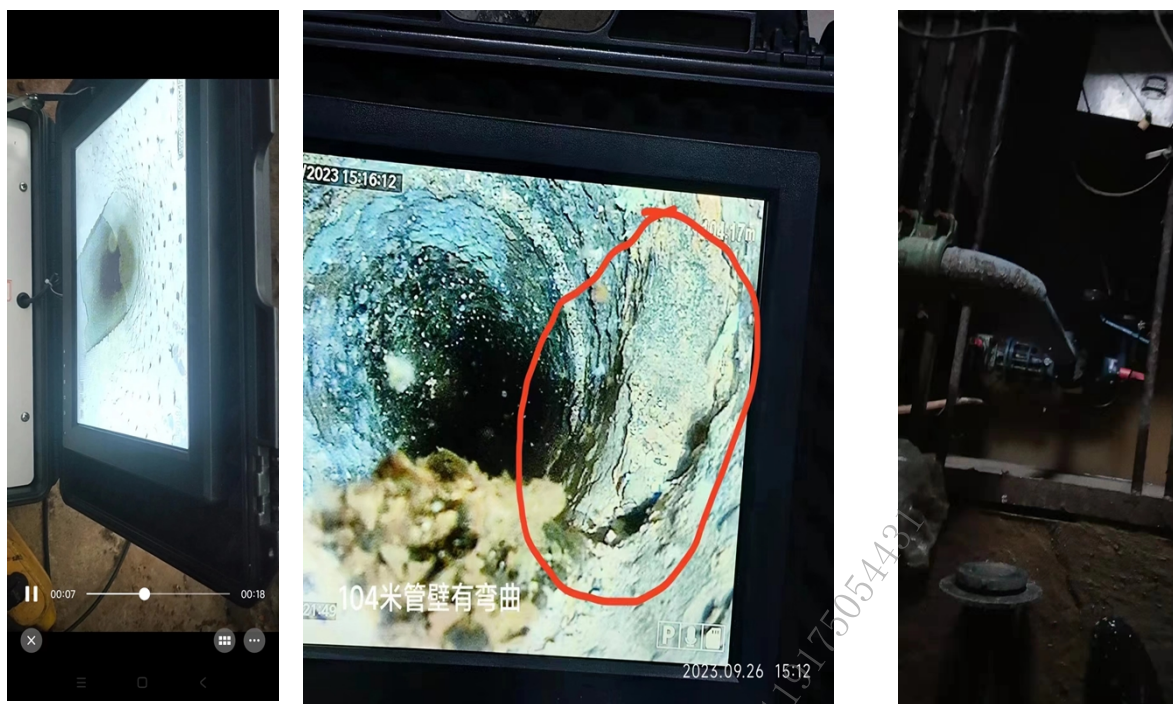
图 3-1 水源井水毁破坏情况
