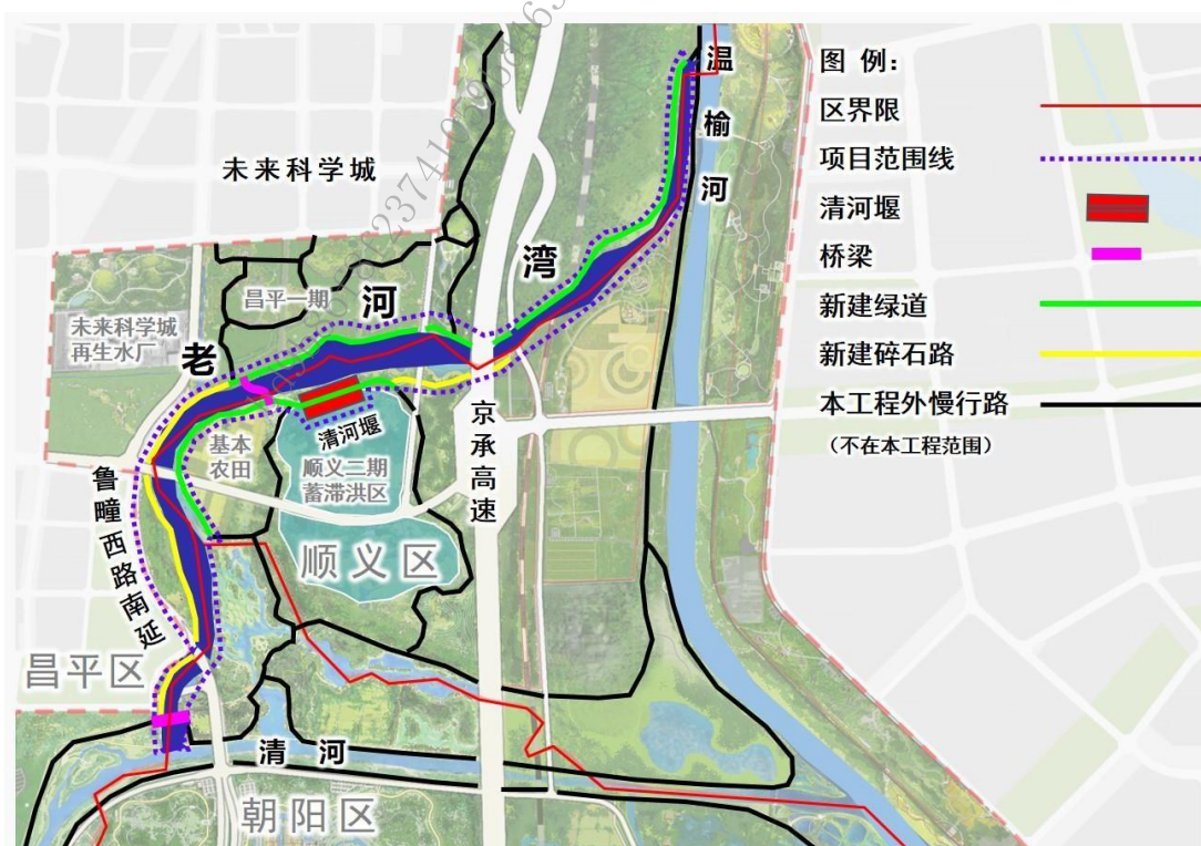
图 1-4 清河老河湾生态治理工程平面布置示意图
