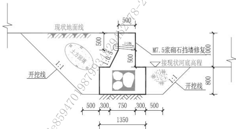
图 5-5 修复损毁 1m 高挡土墙标准设计图二
