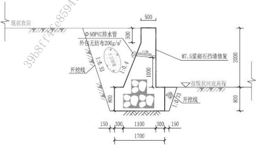
图 5-1 修复 2m 高土挡墙标准设计图
