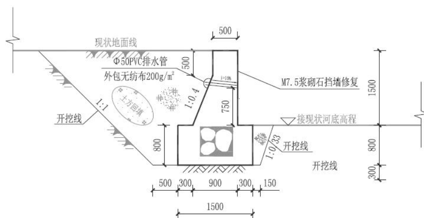
图 5-3 修复 1.5m 高挡土墙标准设计图二
