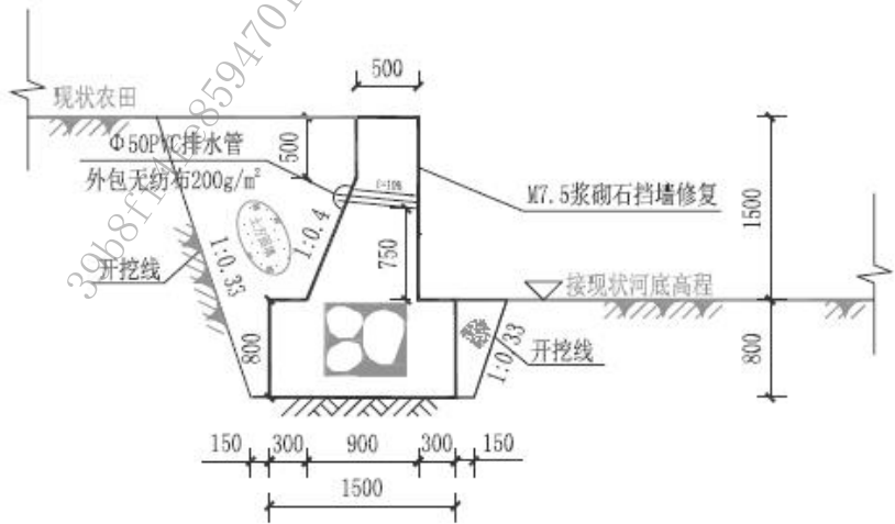
图 5-2 修复 1.5m 高挡土墙标准设计图一
