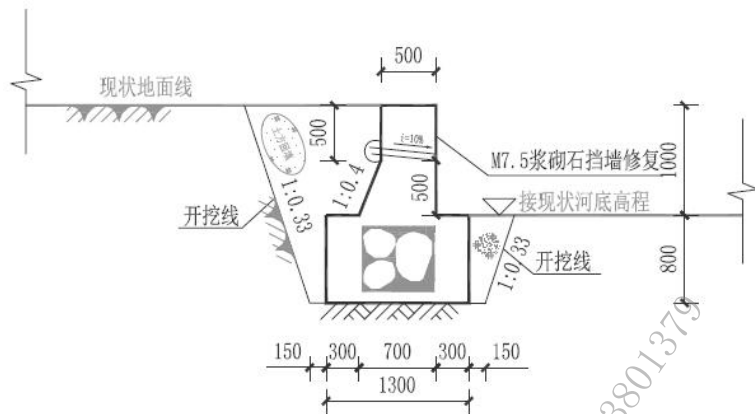
图 5-4 修复损毁 1m 高挡土墙标准设计图一
