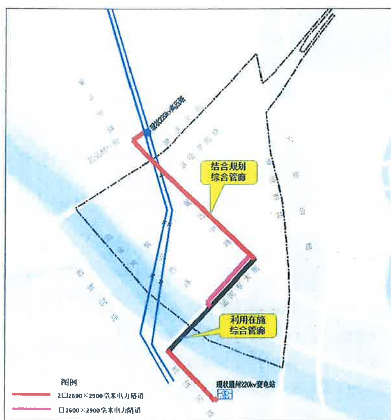
图 9 副中心站综合交通枢纽地区 220 千伏电力迁改方案二示意图
